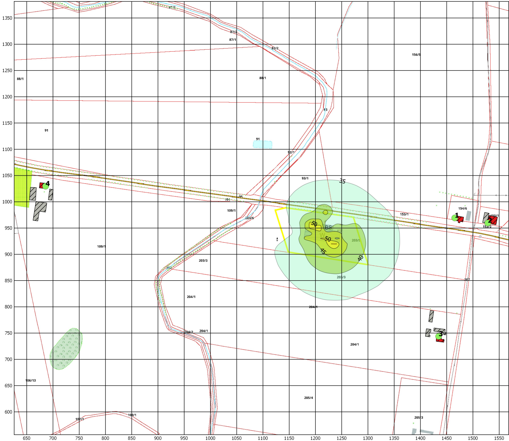
5.1. - Wykres izofon
